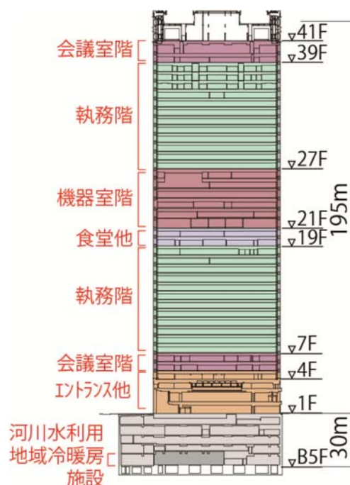
建物断面図
